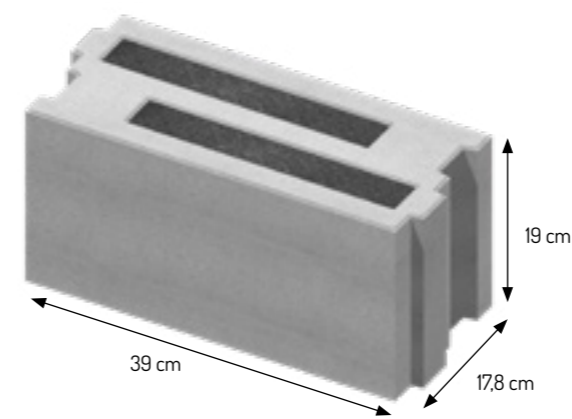
Pustak termiczny 17,8 cm
