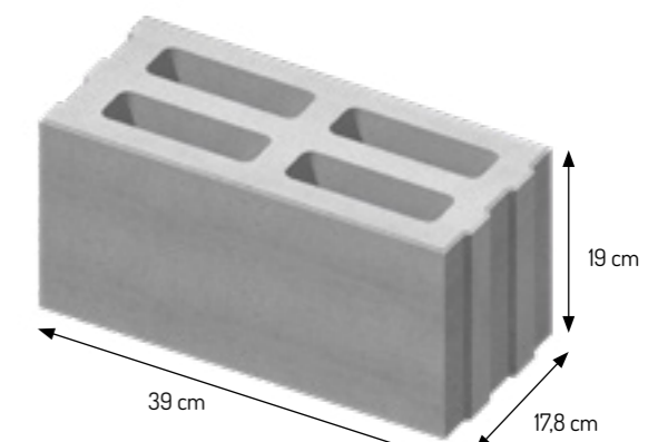
Pustak 17,8 cm
