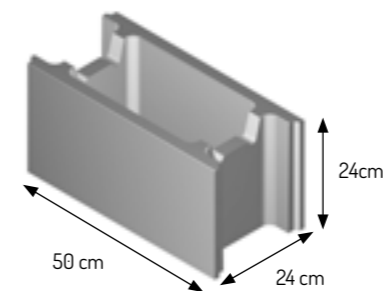
Pustak szalunkowy
