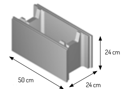
Pustak szalunkowy naprowadzający
