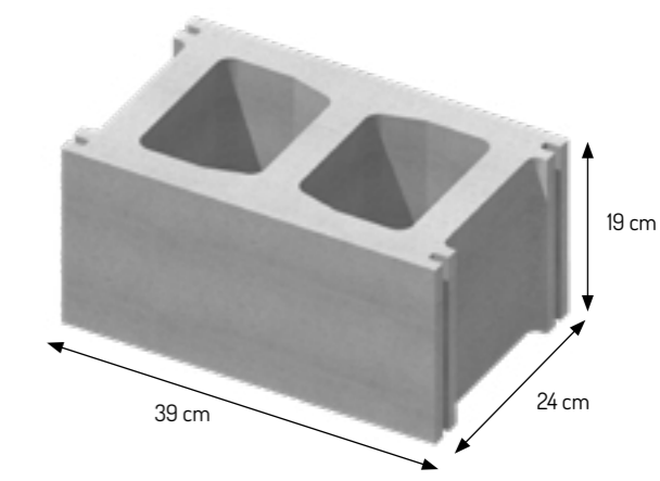
Pustak 24 cm
