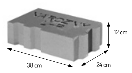
Bloczek P+W narożny
