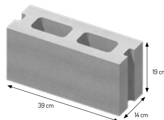
Pustak 14 cm
