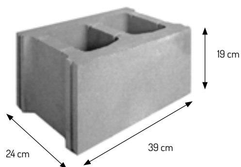
Pustak 24 cm
