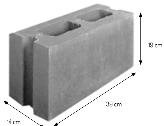
Pustak 14 cm
