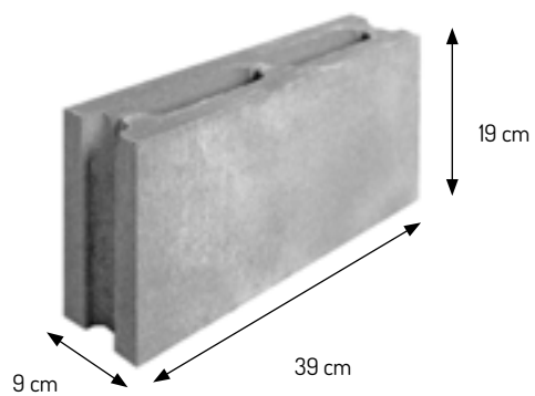
Pustak 9 cm
