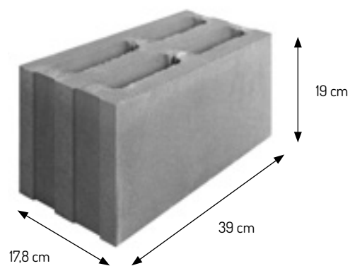
Pustak 17,8 cm
