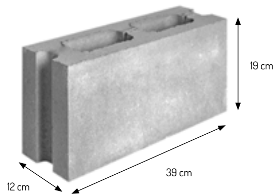
Pustak 12 cm
