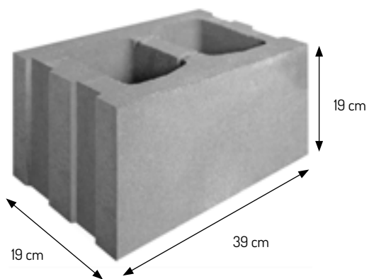
Pustak 19 cm
